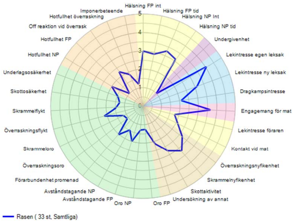
BPH 2007-2016 (33 stycken)
